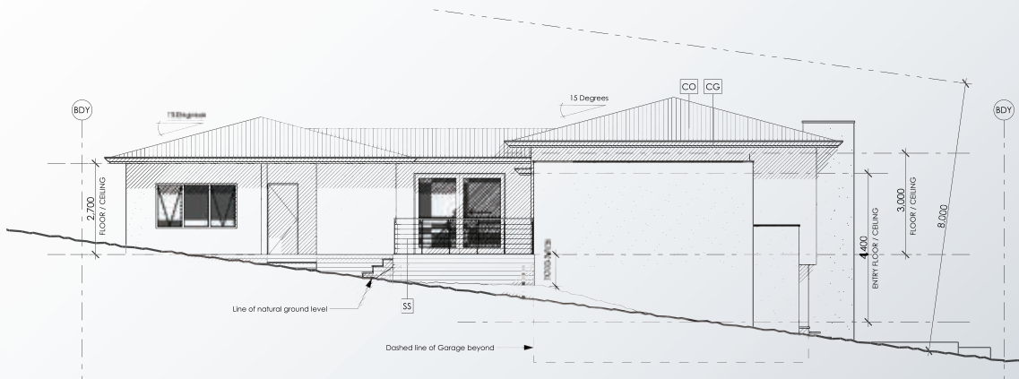
ELEVATION 1:100
